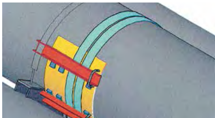
12. ábra – A megerősített külső, meder felőli takarási módszer vázlata
