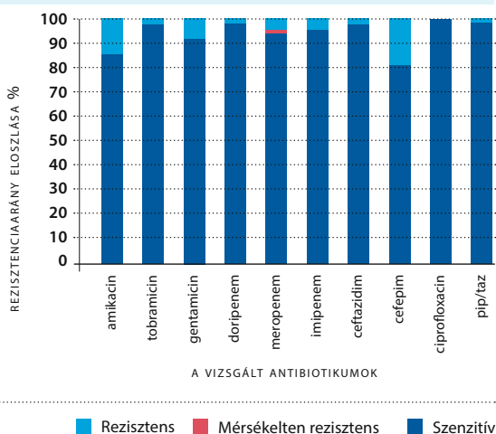
1. ábra Környezeti Pseudomonas aeruginosa izolátumok antibiotikum-rezisztencia profilja
