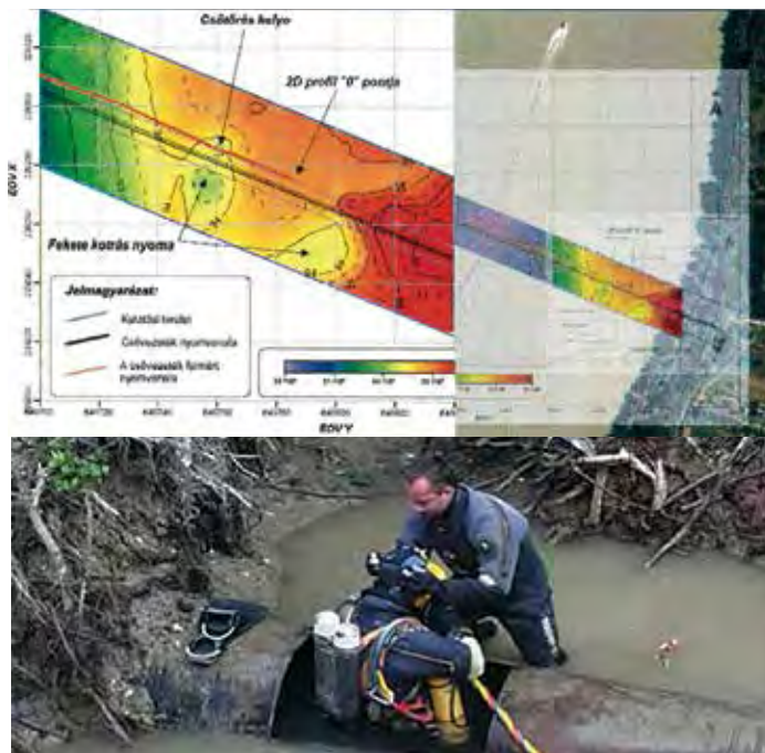
7-8. ábra - Hibahely meghatározás búváros merüléssel a Duna meder alatti DN 1200 mm-es csővezetékben
